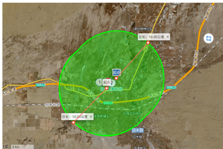
图 1 且末玉都机场飞行区电磁环境保护区域
