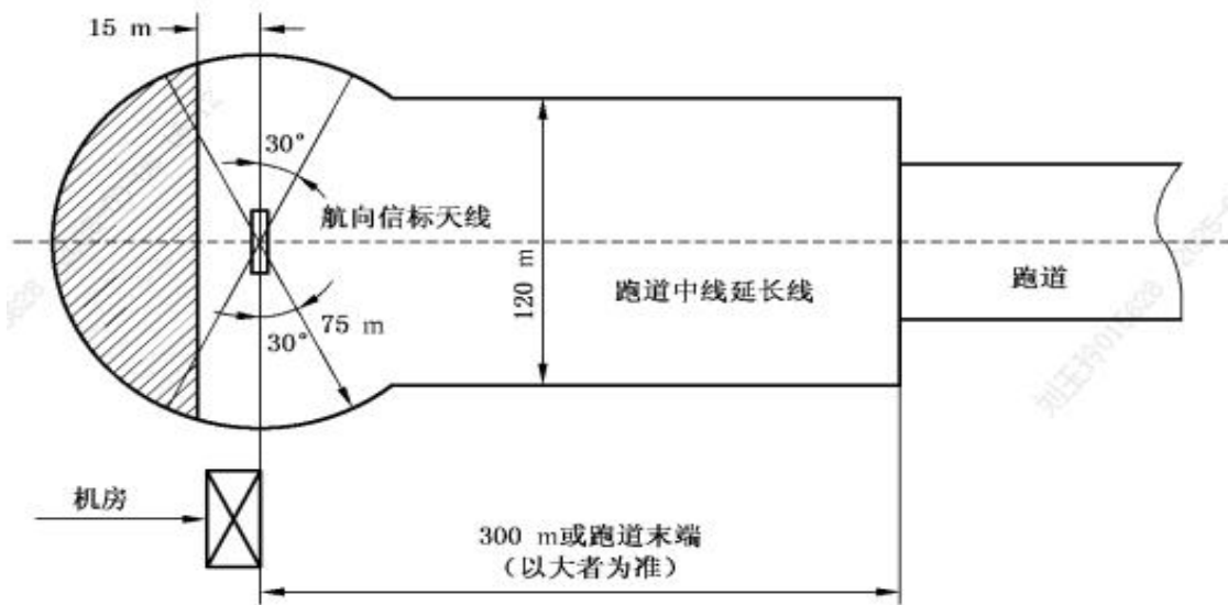
图 3 航向信标台保护区
